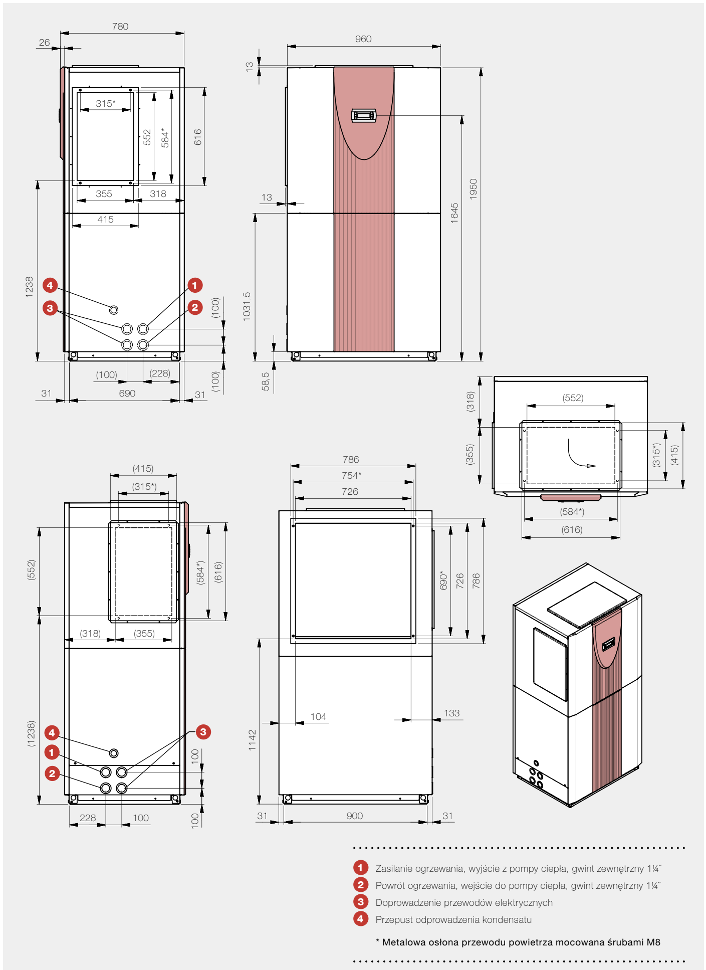
Rysunek wymiarowy
